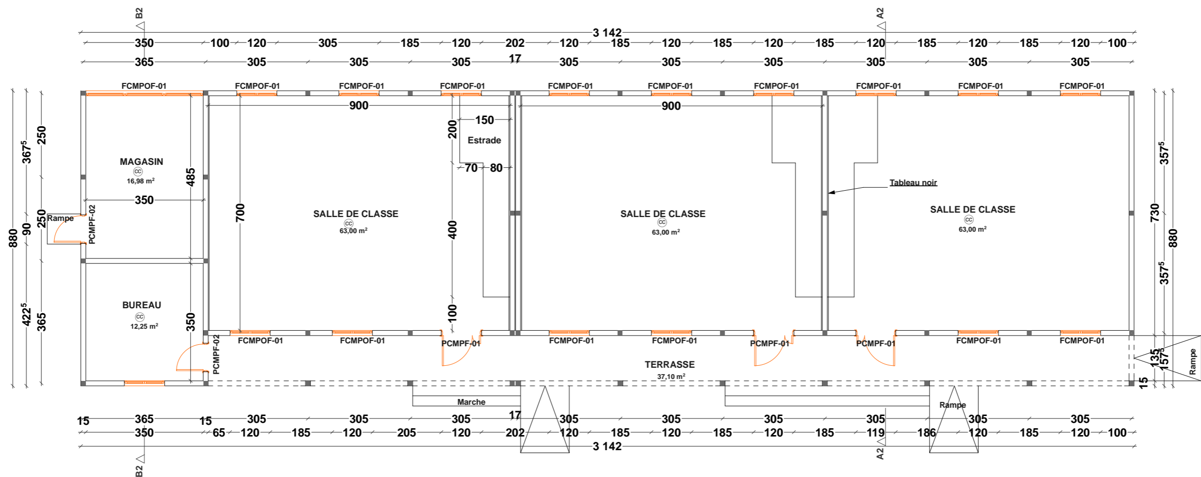
PLAN DE NIVEAU
