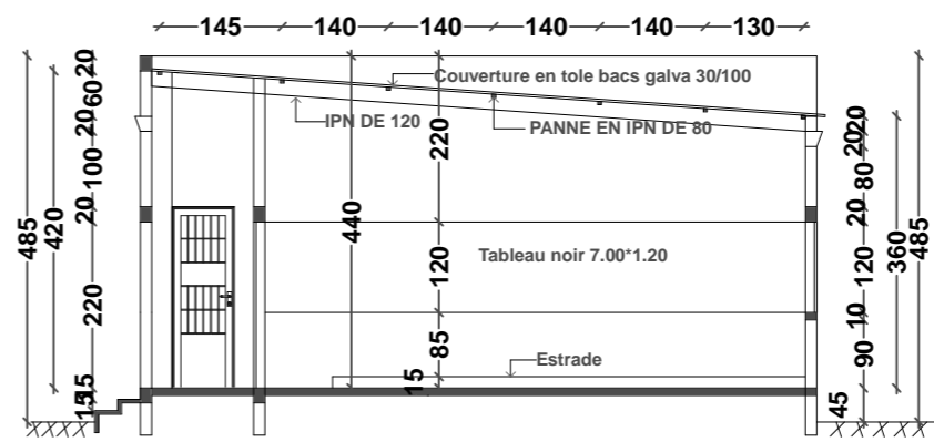
COUPE A-A
