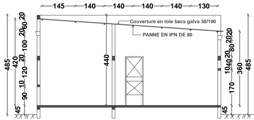
COUPE B-B
